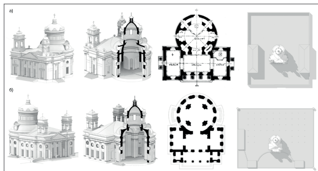
Рис. 2. Церковь Сошествия Св. Духа на Лазаревском кладбище в Москве (общий вид, аксонометрический открытый разрез, план и генплан): а) Реконструкция первоначального замысла по проекту Н. Леграна; б) Реконструкция церкви на период строительства Е. С. Назаровым. Научно-графическая реконструкция выполнена студ. МАРХИ М. А. Барковой и А. И. Солдатовой, науч. рук. Ю. Г. Клименко
