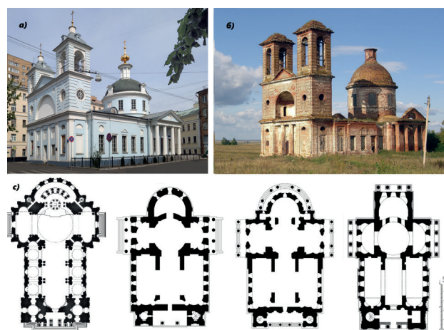
Рис. 3. Двухколоколенные храмы конца XVIII – начала XIX в.: а) Церковь Успения Пресвятой Богородицы на Могильцах. Москва. Фото автора; б) Церковь Архангела Михаила в с. Порошино (Пензенская обл.). Фото автора; в) Сравнительный анализ планов: - Троицкий собор Александро-Невской лавры. Санкт-Петербург; - Церковь Успения на Могильцах. Москва; - Церковь Сошествия Св. Духа в с. Шкинью. 1794–1800-е гг. (Московская обл.); - Церковь Архангела Михаила в с. Порошино (Пензенская обл.)
