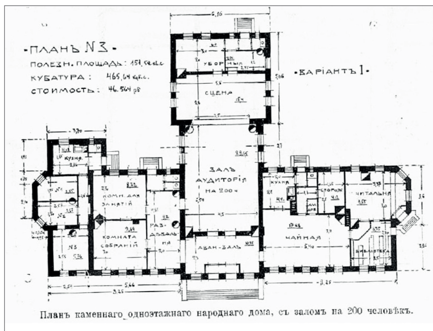
Рис. 3. План № 3, вариант 1. План каменного одноэтажного Народного дома с залом на 200 человек
