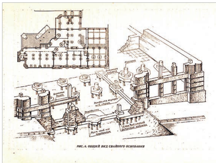
Рис. 2. Изображение свайного основания здания и его план из книги «Архитектурные конструкции» [2, с. 35]
