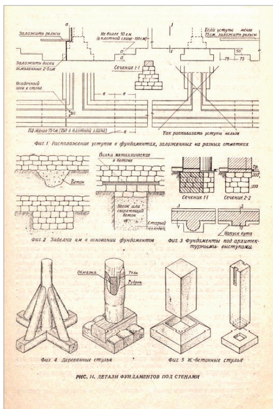
Рис. 3. Чертежи из книги «Архитектурные конструкции»:
